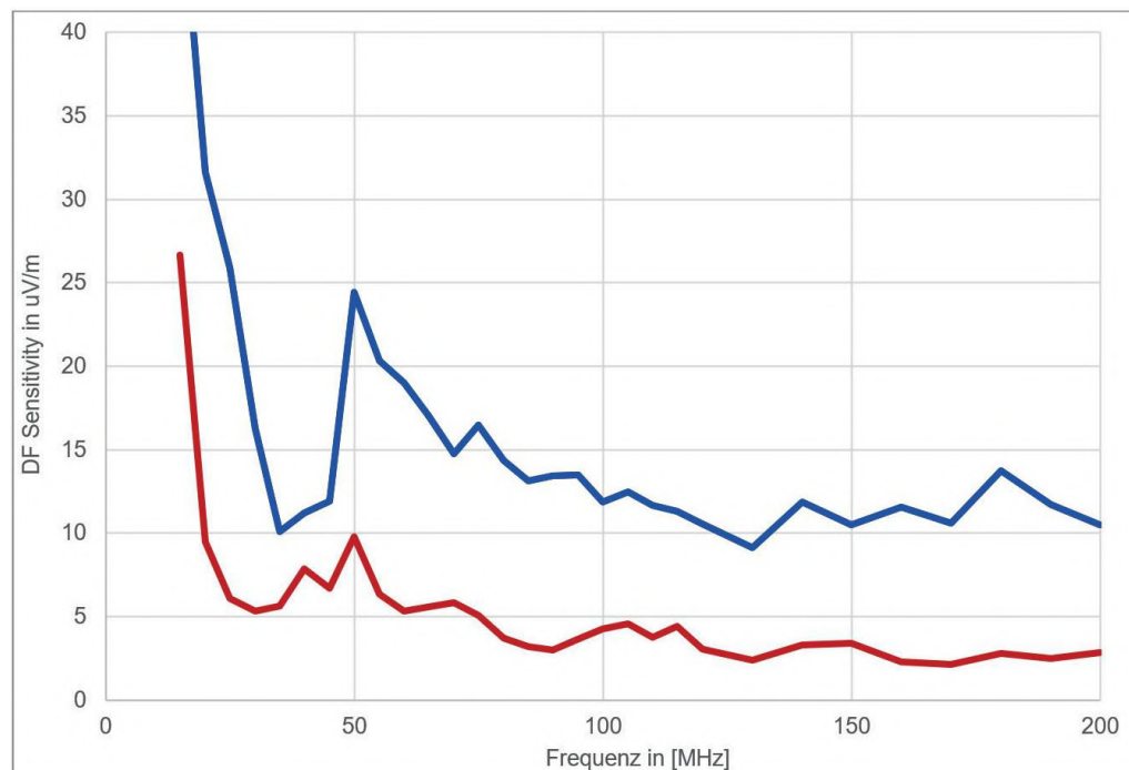
図12 : ITU-R SM.2096-0に準じた3° RMS方位変動時のDF感度
