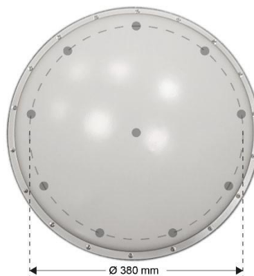
図2：大きな開口部：9つのダイポールエレメントで高いDF確度を実現
