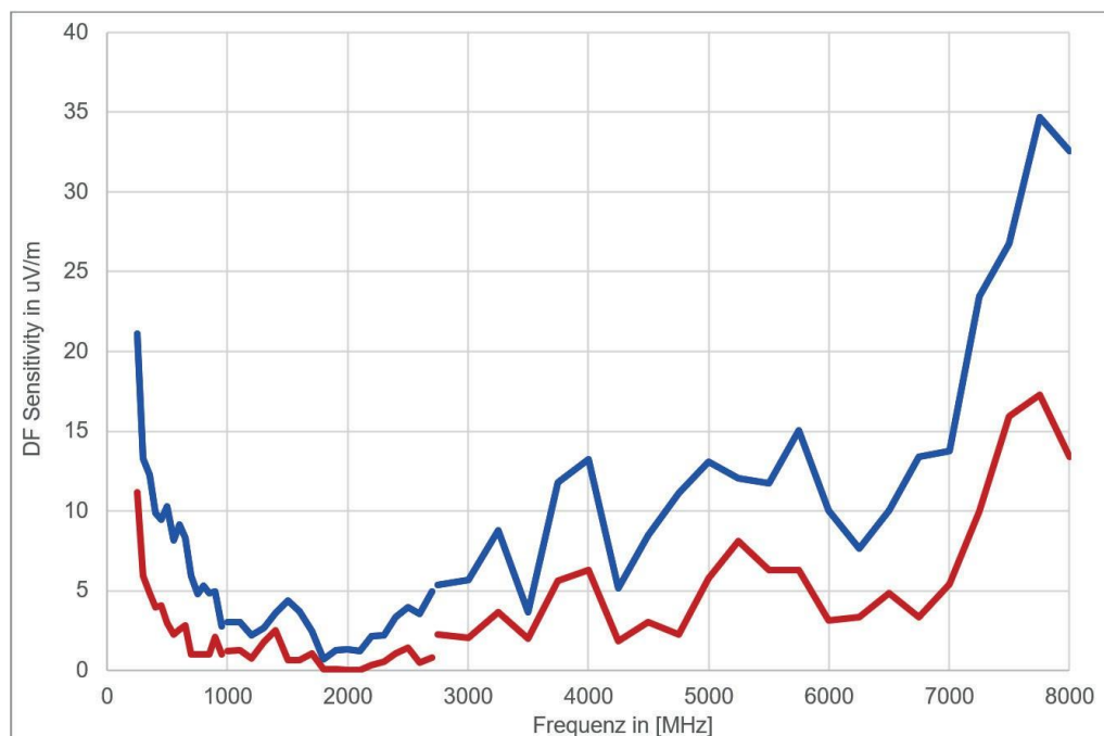
図13 : ITU-R SM.2096-0に準じた3° RMS方位変動時のDF感度
